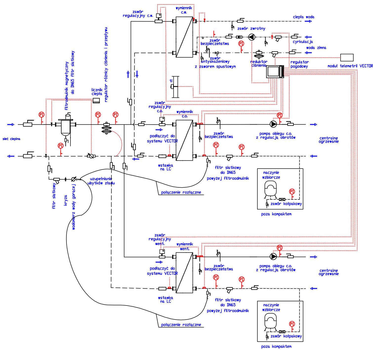
Załącznik nr 5 SCHEMAT TECHNOLOGICZNY WĘZŁA CIEPLNEGO C.O. + WENT. + C.W. JEDNOSTOPNIOWEGO finansowanego przez Veolia Energia Poznań S.A.
